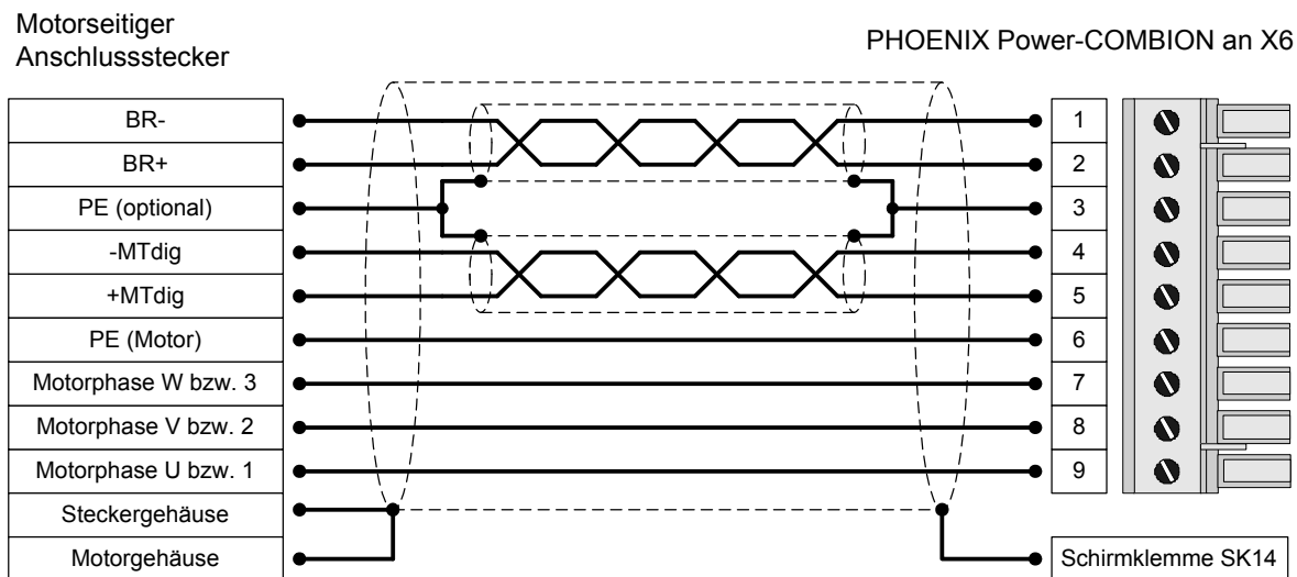
Abbildung 19: Motoranschluss [X6]
