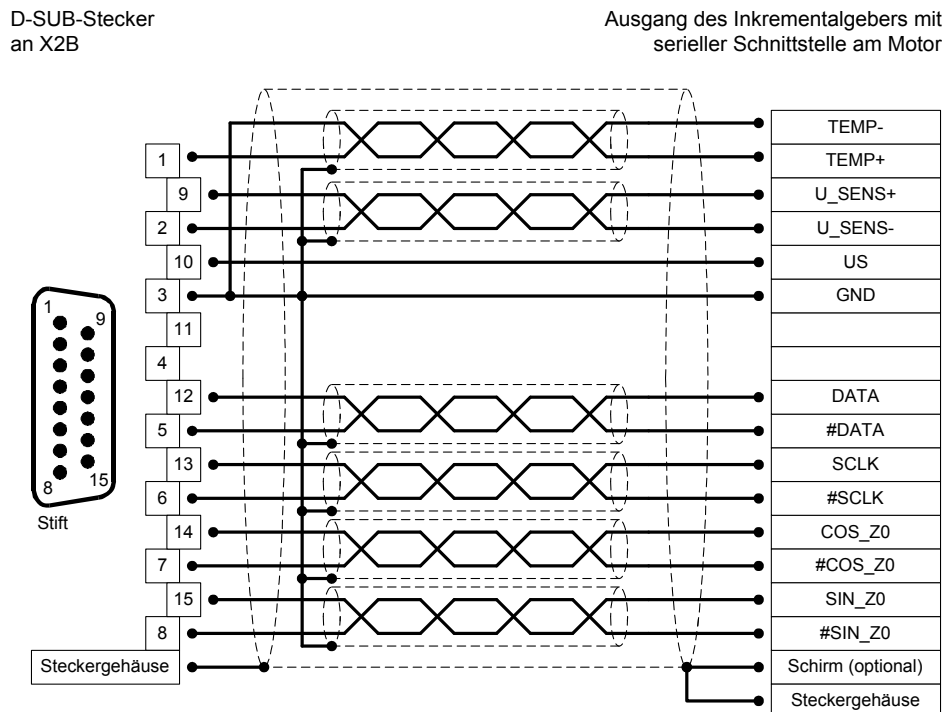
Abbildung 25: Steckerbelegung: Inkrementalgeber mit serieller Schnittstelle (z.B. EnDat, HIPERFACE) – optional [X2B]
