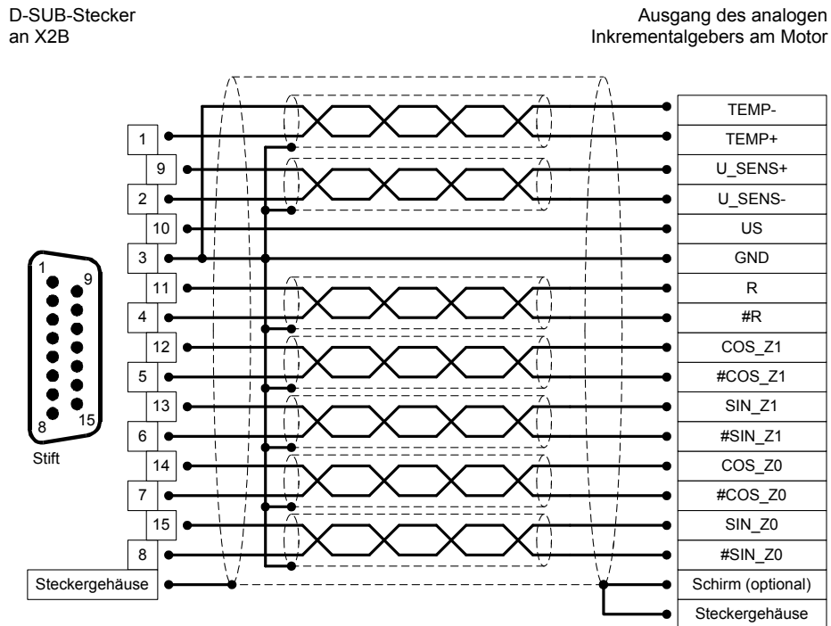
Abbildung 24: Steckerbelegung: Analoger Inkrementalgeber – optional [X2B]
