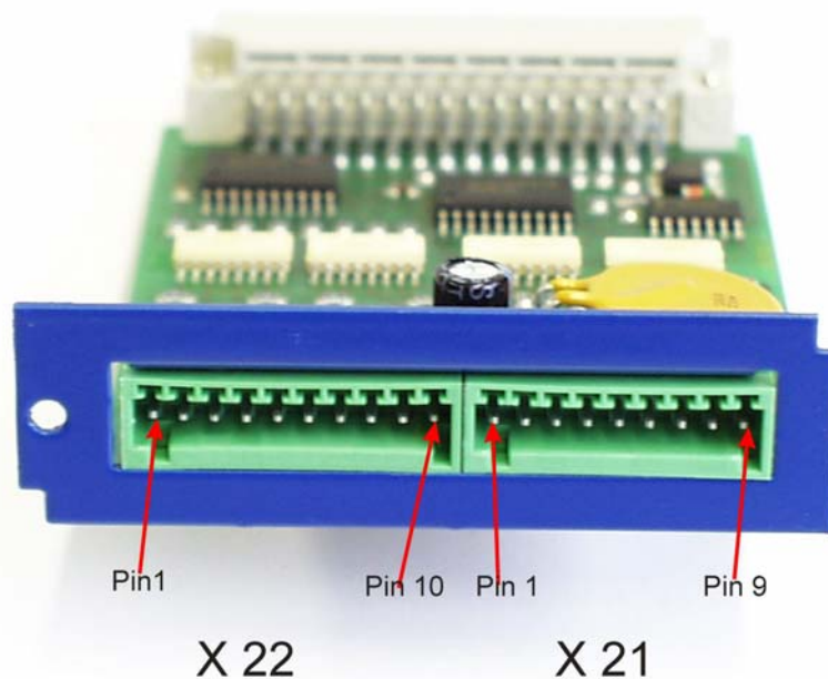
Abbildung 34: EA88: Lage der Steckverbinder [X21] und [X22] an der Frontplatte
