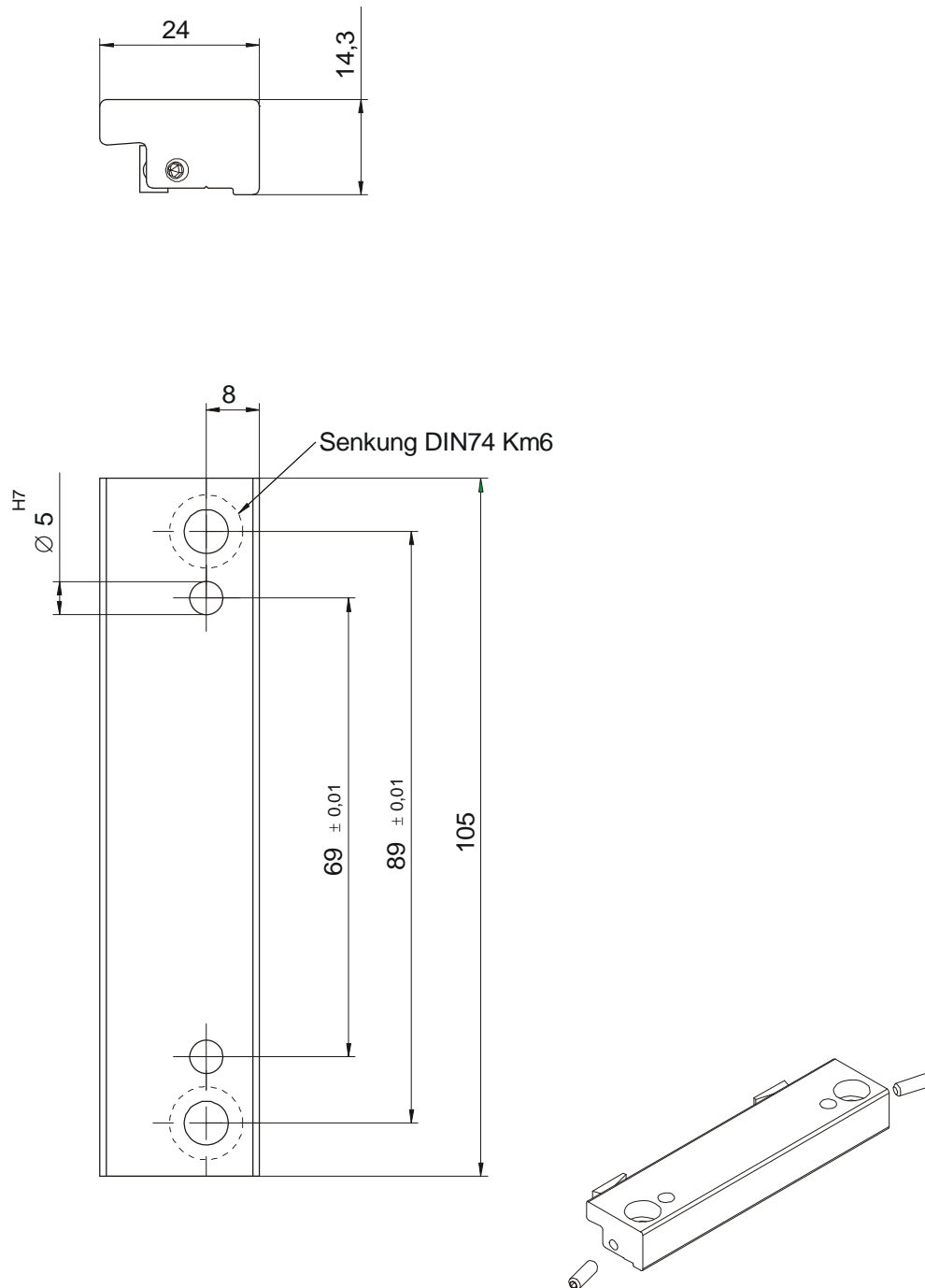
Abbildung 21: Spannelement 526607
