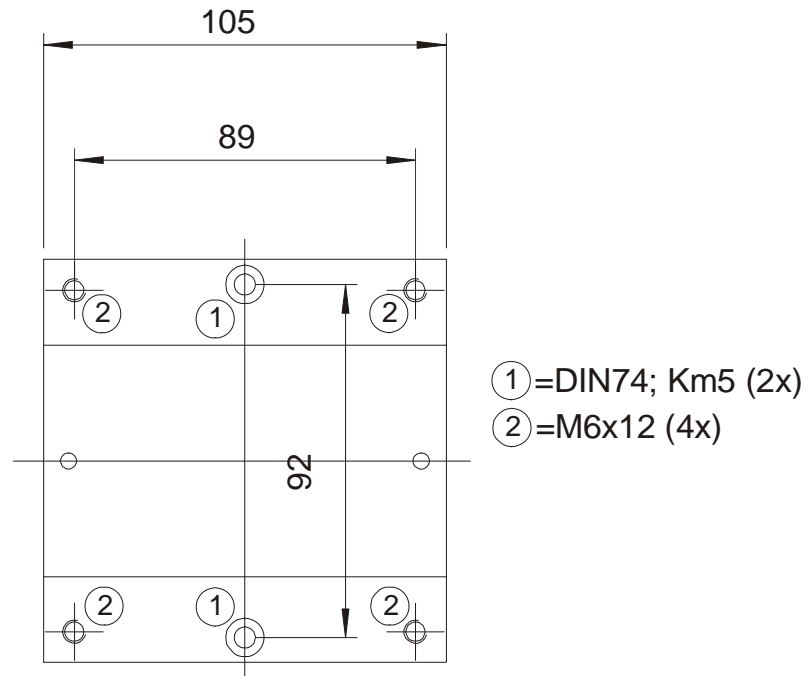
Abbildung 4: Schlittenbohrbild
