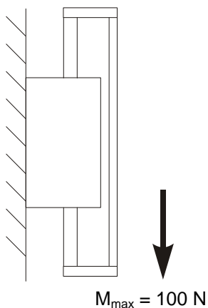
Abbildung 10: Maximale Belastung
